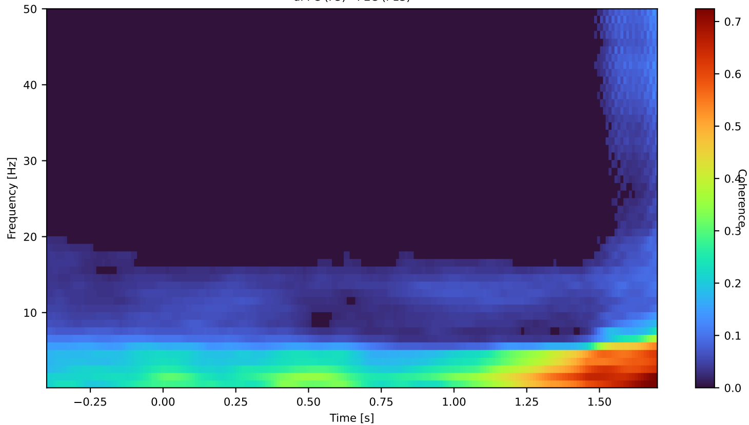
dPFC (F5) - PEC (P13)
